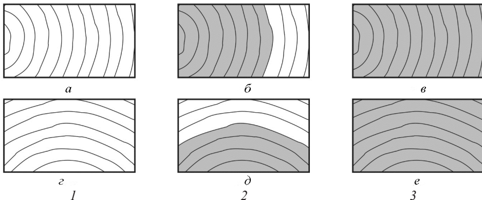
Рис. 2. Группы образцов по типу древесины и расположению слоев: 1 – заболонная древесина; 2 – смешанная (ядровая заболонная) древесина; 3 – ядровая древесина; а, б, в – с радиальным расположением слоев; г, д, е – с тангенциальным
