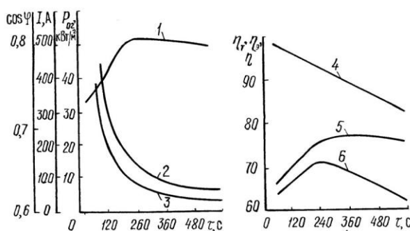
Изменение коэффициента мощности \cos \varphi (1), удельной поверхностной мощности P_{02} (2), тока индуктора I (3), теплового \eta_T (4), электрического \eta_e (5) и полного \eta (6) КПД в зависимости от времени \tau (напряжение на индукторе 73 В)
